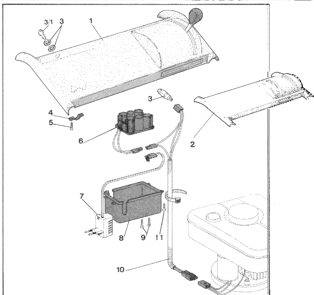
KIT AVVIAMENTO ELETTRICO mod. 943/CV/K - mod. 943/CSV/K - mod. 948/CSV/K
