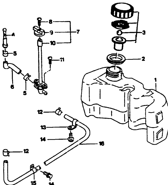
Tank FC 150 V - ES 63, ES 64
